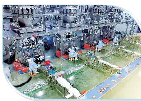
鹿邑县丸来丸去有限公司牛肉丸制品智能化生产线改造项目。
